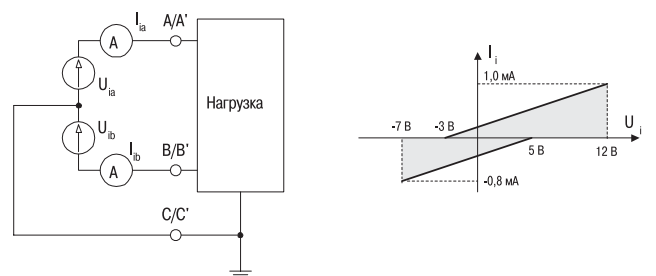
Нагрузкой является совокупность приемника и формирователя, переведенного в пассивное состояние.
