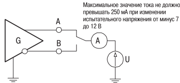
Рис. 10. Схема проверки формирователя в условиях возникновения конфликтных ситуаций
