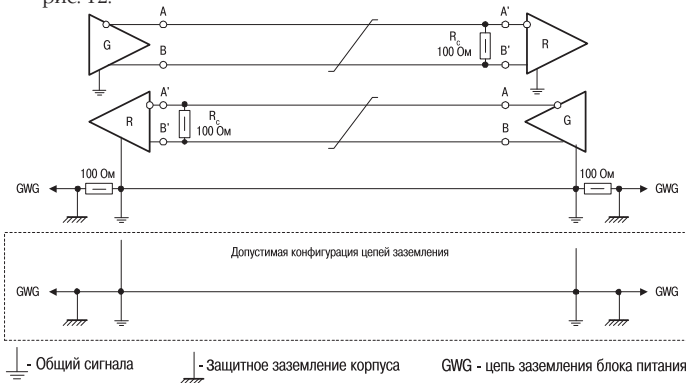
Рис. 12. Основная конфигурация системы связи на базе передатчиков, соответствующих требованиям EIA RS-422A
