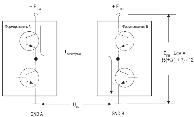
Рис. 18. Конфликтная ситуация, вызванная одновременной активизацией двух формирователей
